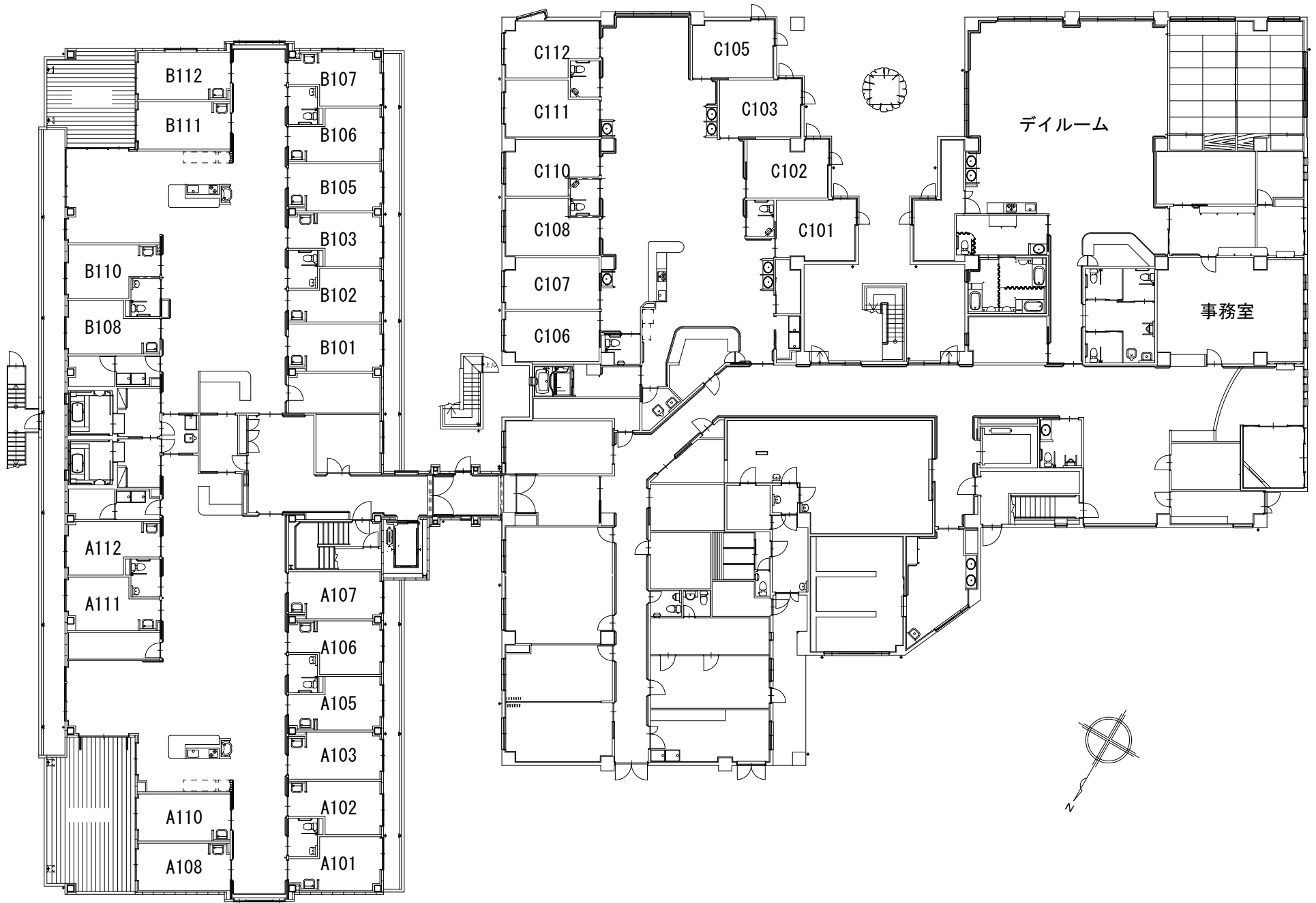
1 階 平 面 図
